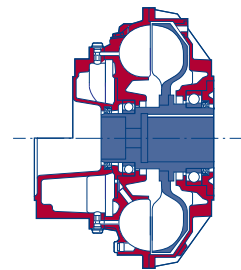
Type TVV
